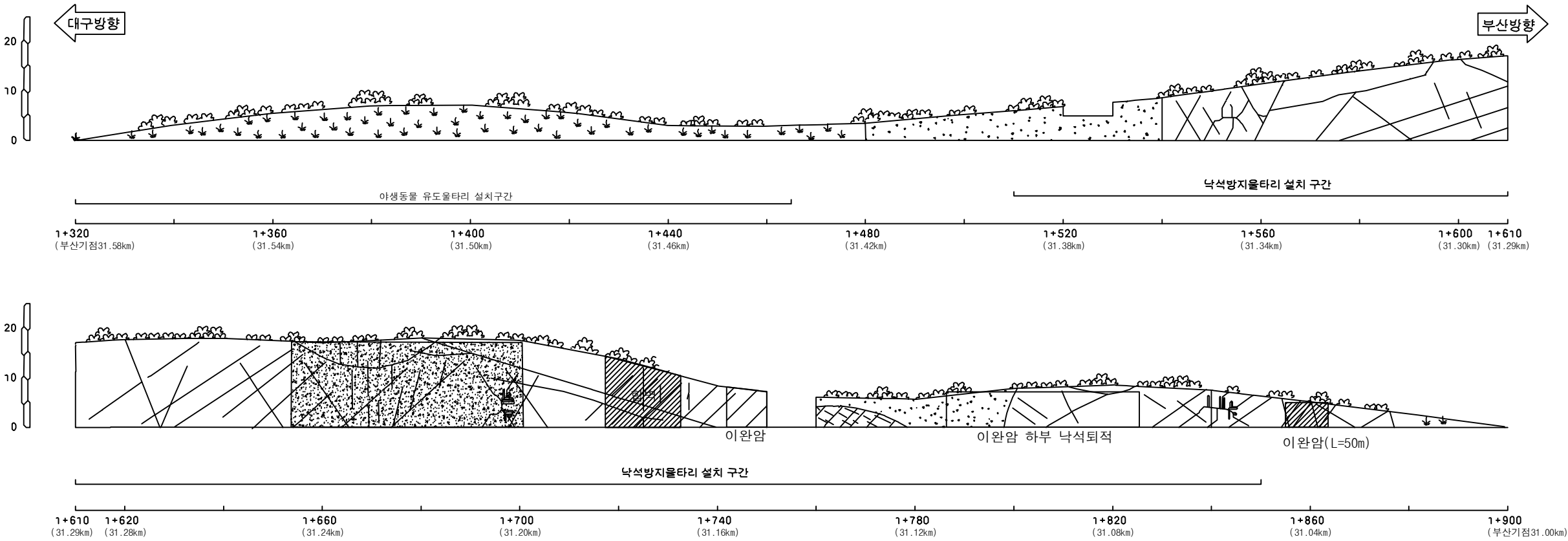
부산기점 31.00~31.58km (9공구 STA.1+320~1+900)
