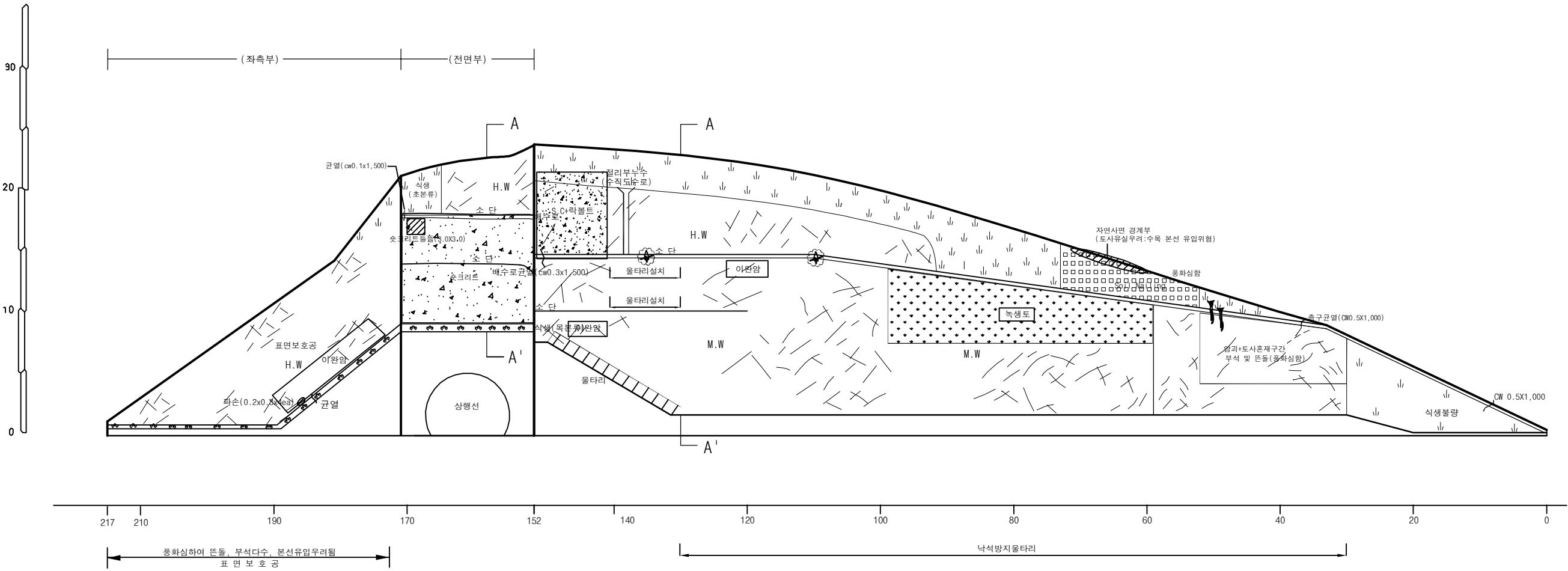
부산기점 17.60km (10공구 STA4+060), 상동2터널 시점부 상행선
