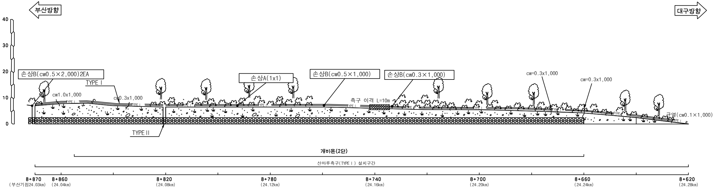
부산기점 24.03~24.28km (9공구 STA.8+620~8+870)
