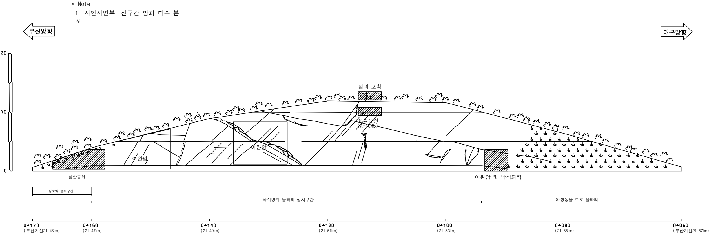
부산기점 21.46~21.57km (10공구 STA.0+060~0+170)
