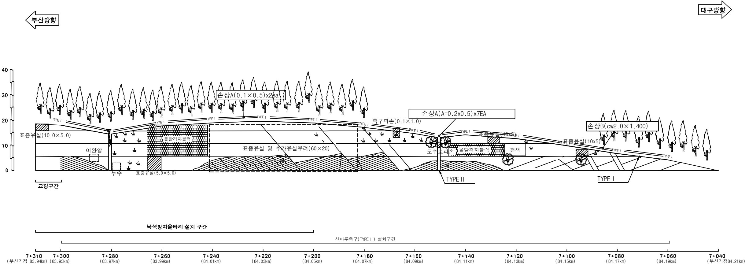
부산기점 83.94~84.21km (2공구 STA.7+040~7+310)
