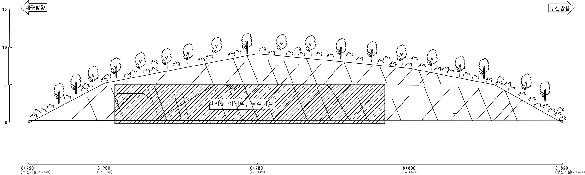
부산기점 67.64~67.71km (4공구 STA.8+750~8+820)
