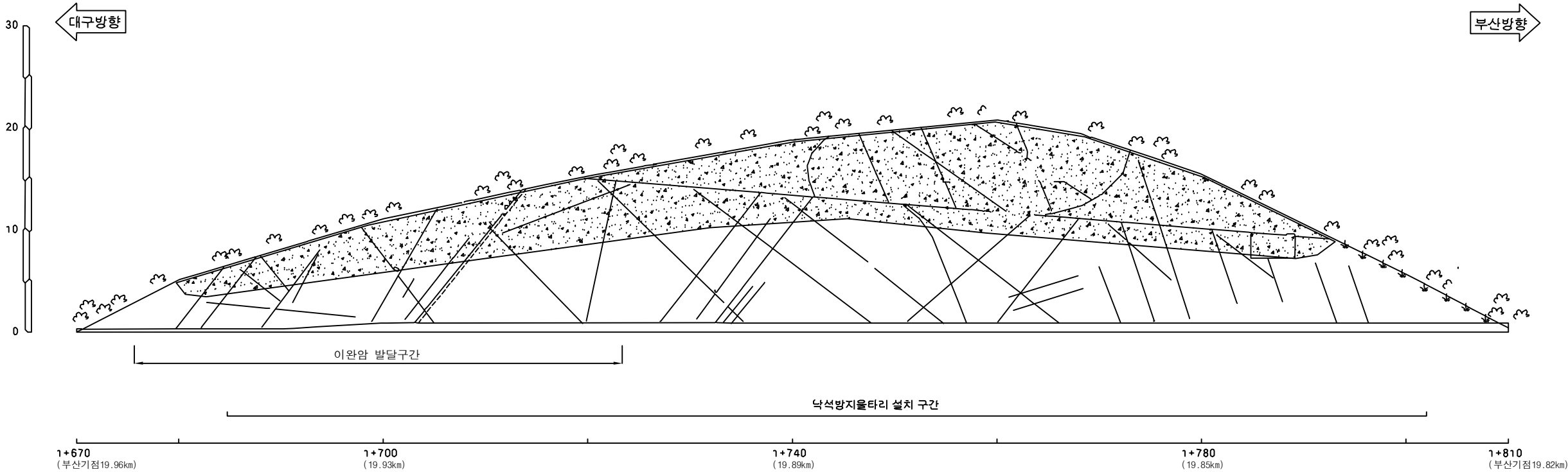
부산기점 19.82~19.96km (10공구 STA.1+670~1+810)
