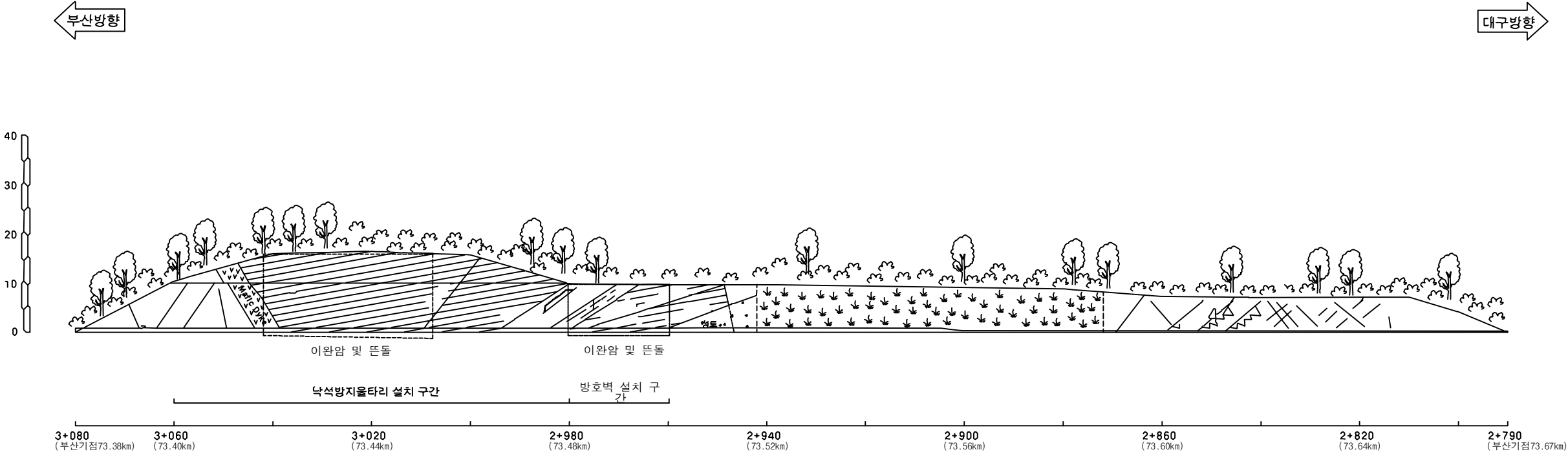
부산기점 73.38~73.67km (4공구 STA.2+790~3+080)
