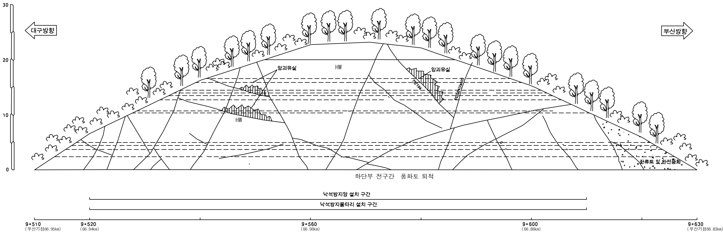
부산기점 66.83~66.95km (4공구 STA.9+510~9+630)
