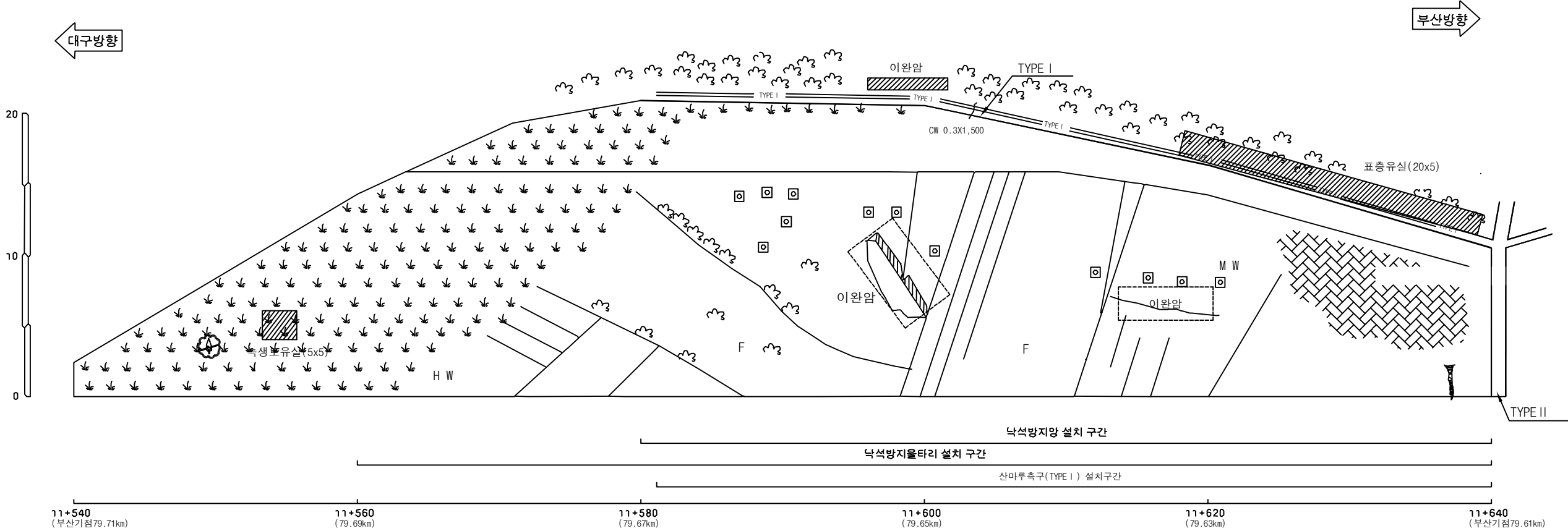
부산지점 79.61~79.71km (3공구 STA.11+540~11+640)
