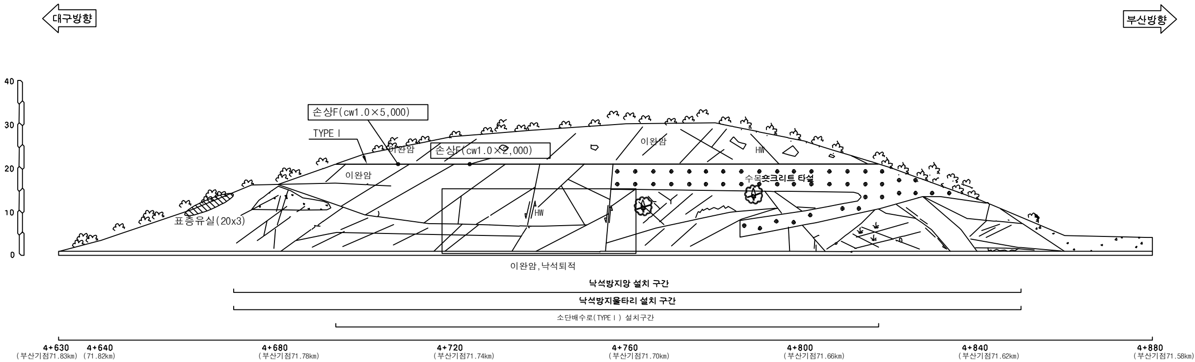
부산기점 71.58~71.83km (4공구 STA.4+630~4+880)
