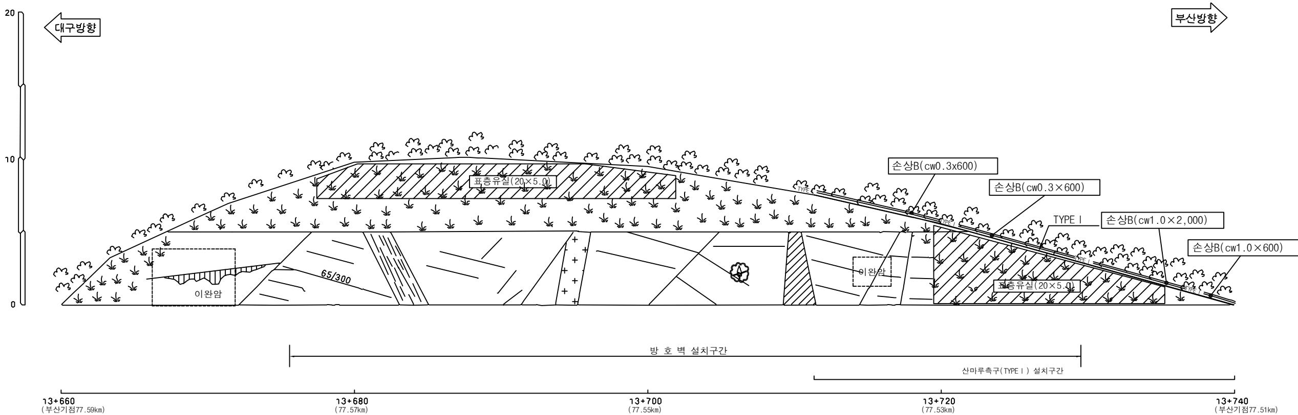
부산지점 77.51~77.59km (3공구 STA.13+660~13+740)
