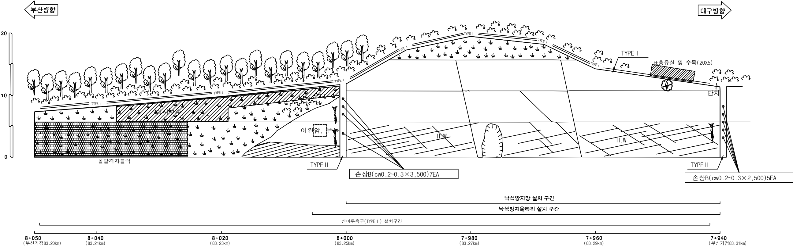
부산기점 83.20~83.31km (2공구 STA.7+940~8+050)
