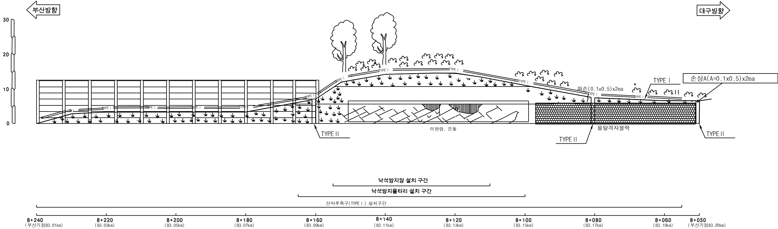
부산기점 83.01~83.20km (2공구 STA.8+050~8+240)
