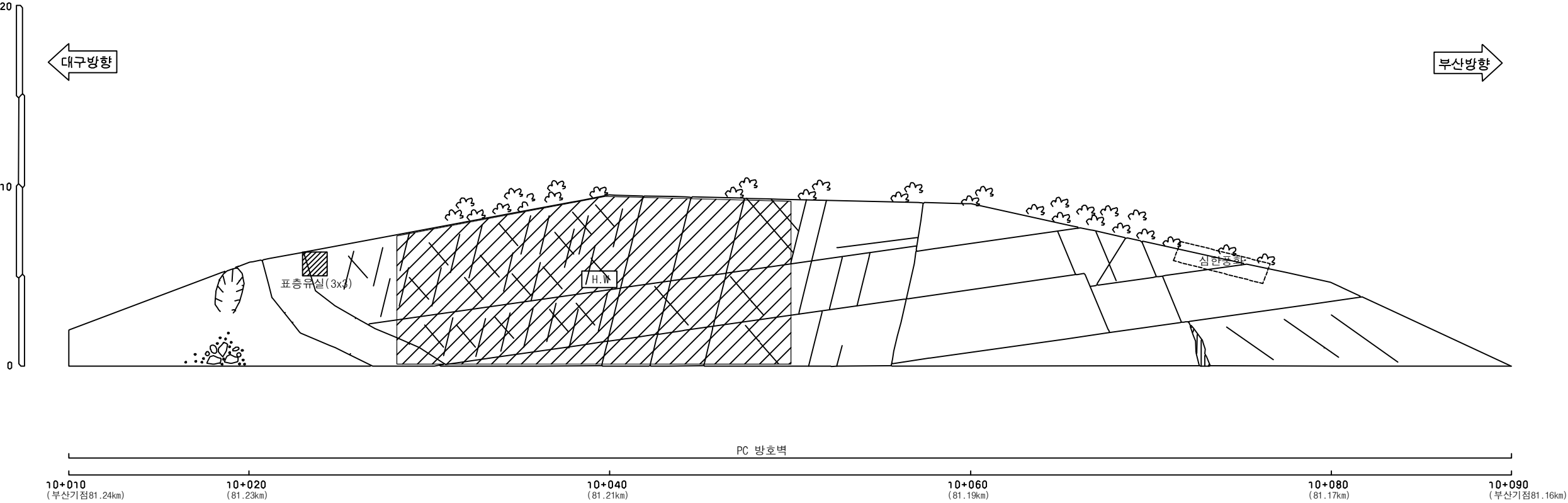
부산기점 81.16~81.24km (3공구 STA.10+010~10+090)
