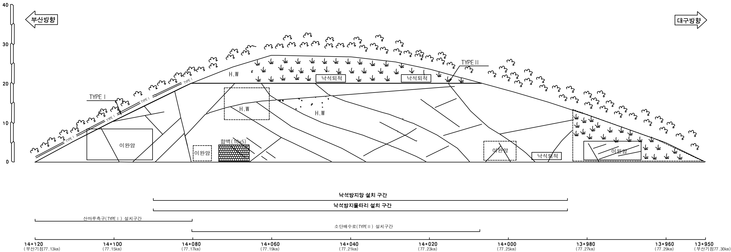
낙석방지망 설치 구간 낙석방지울타리 설치 구간 산마루측구(TYPE I) 설치구간 소단배수로(TYPE II) 설치구간 14+120 (부산기점77.13km) 14+100 (77.15km) 14+080 (77.17km) 14+060 (77.19km) 14+040 (77.21km) 14+020 (77.23km) 14+000 (77.25km) 13+980 (77.27km) 13+960 (77.29km) 13+950 (부산기점77.30km) 부산기점 77.13~77.30km (3공구 STA.13+950~14+120)
