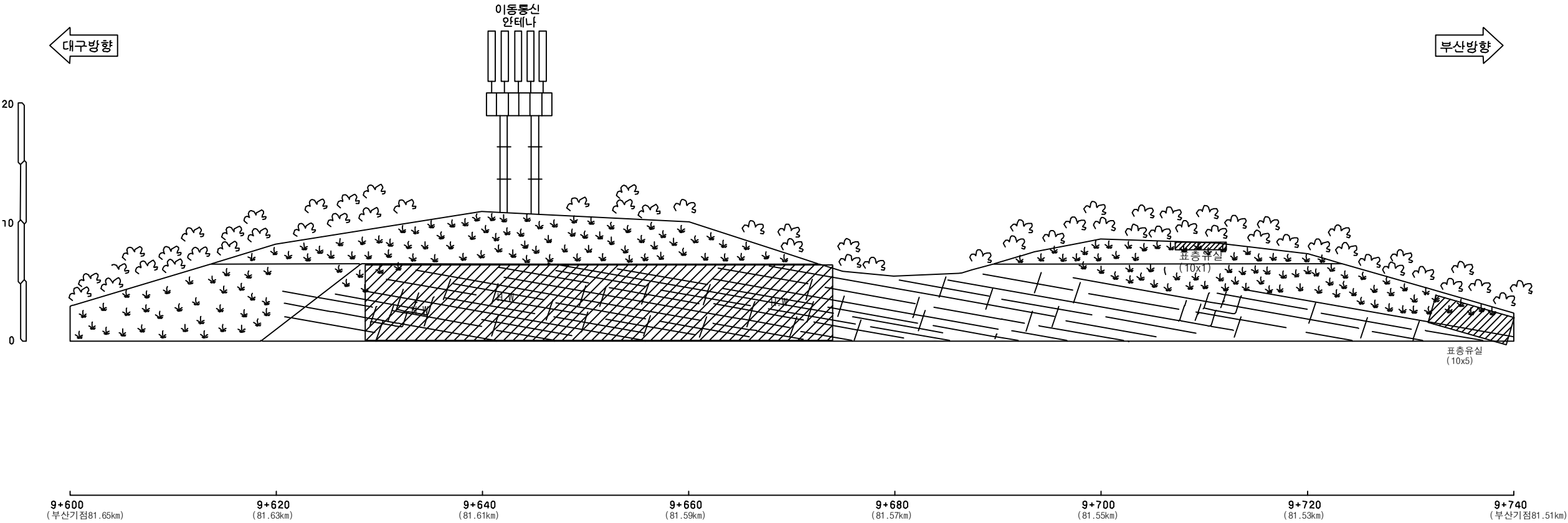
부산기점 81.51~81.65km (3공구 STA.9+600~9+740)
