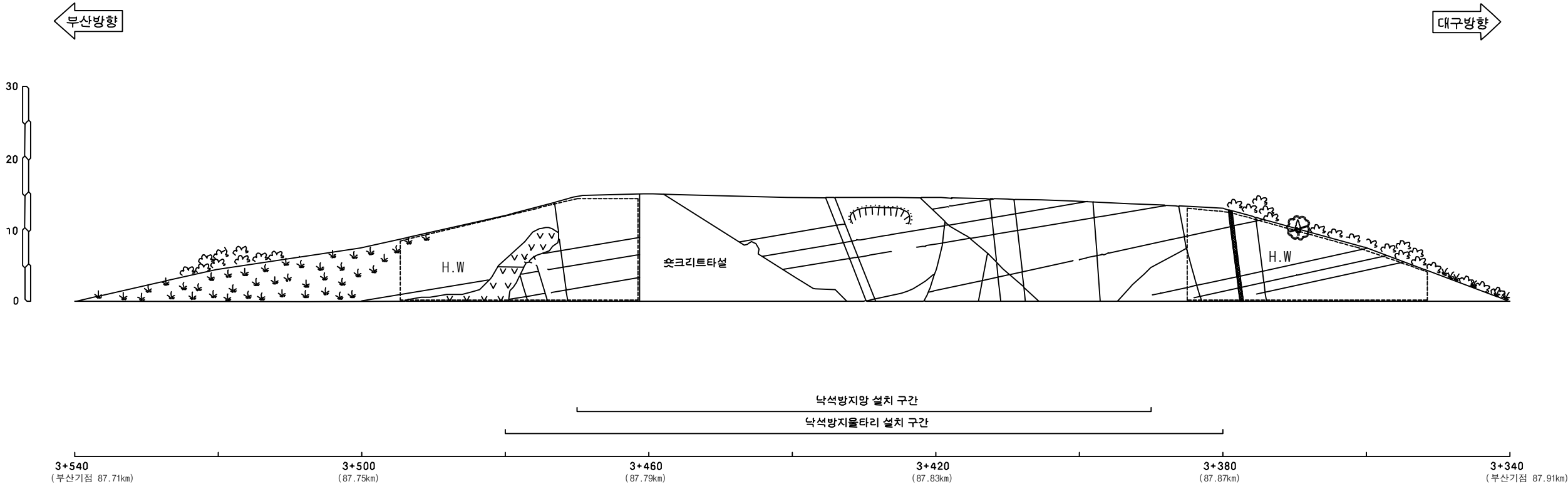
부산기점 87.71~87.91km (1공구 STA.3+540~3+340)
